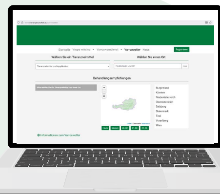
Abbildung 7: Varroawetter: www.bienengesundheit.at/varroawetter
